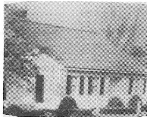
(d) Intensity
