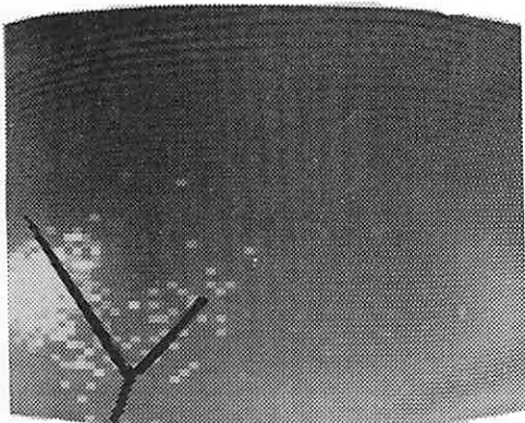
(d) Cluster 4
